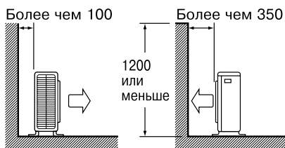
Вид сбоку
