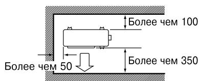
Вид сверху
