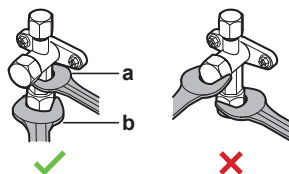
a Гаечный ключ b Динамометрический ключ
