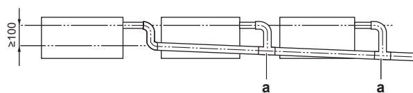
a Тройник
