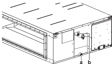
a Подсоединение сливной трубки b Трубопровод хладагента
