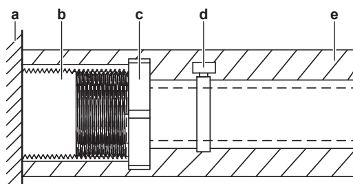
a Внутренний блок b Стандартная трубная внутренняя резьба 1" c Переходник (приобретается по месту установки) d Металлический зажим (приобретается по месту установки) e Изоляционный материал для сливного трубопровода (приобретается по месту установки)
