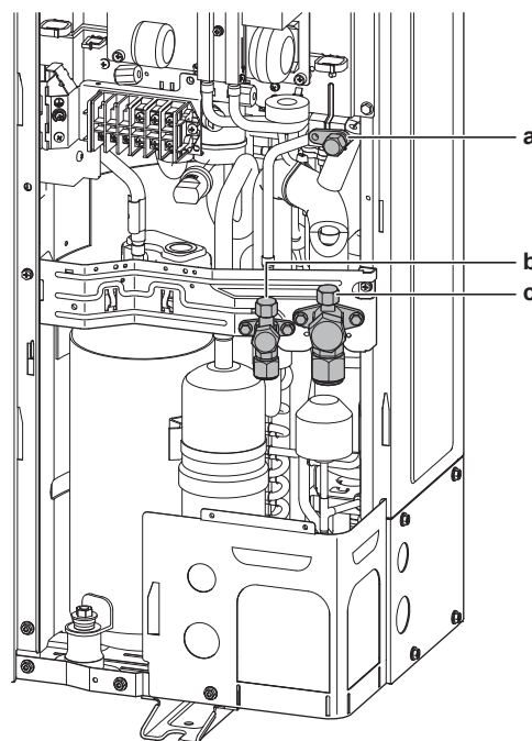
a Внутреннее сервисное отверстие
